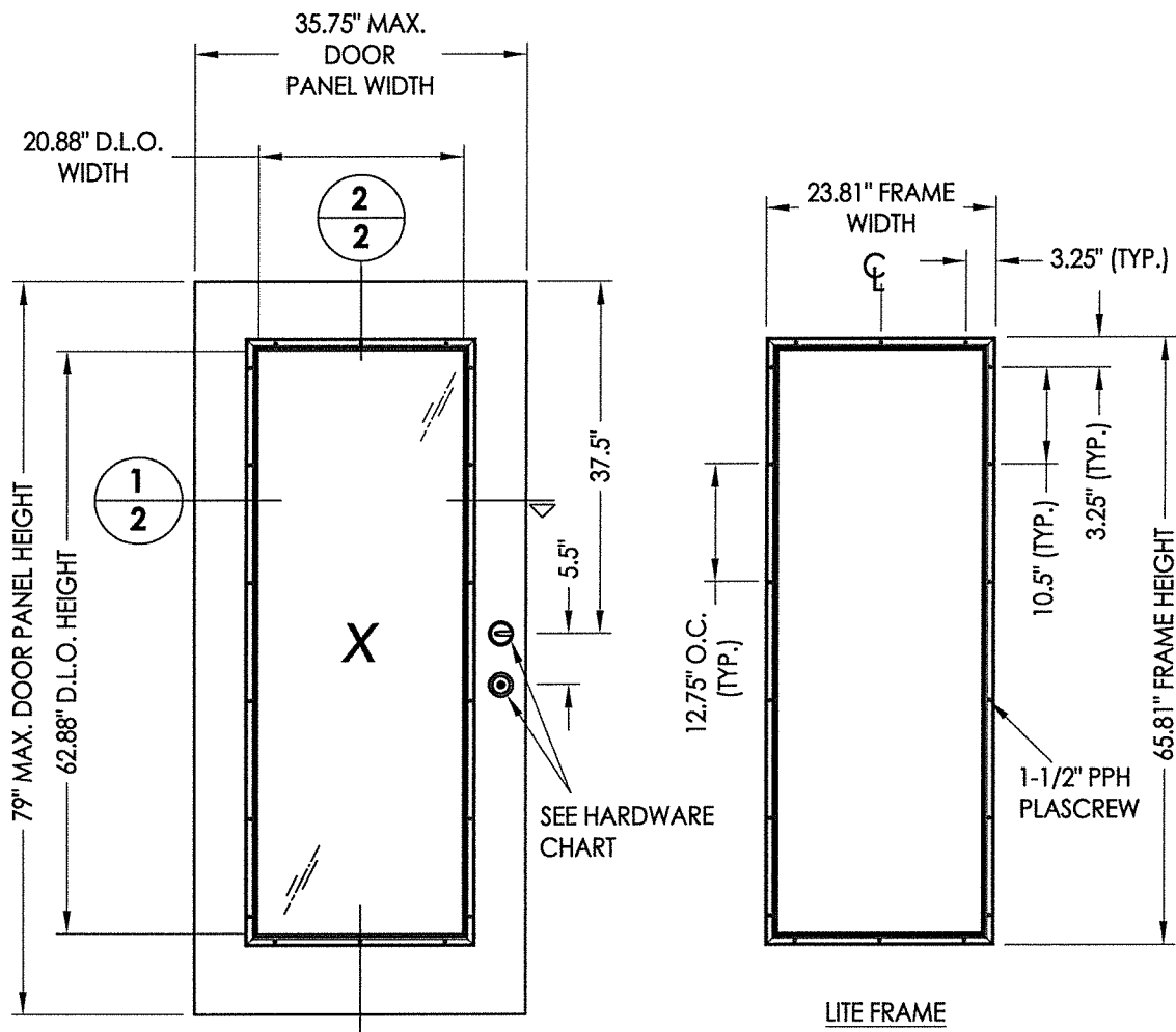
40 DOOR PANEL
