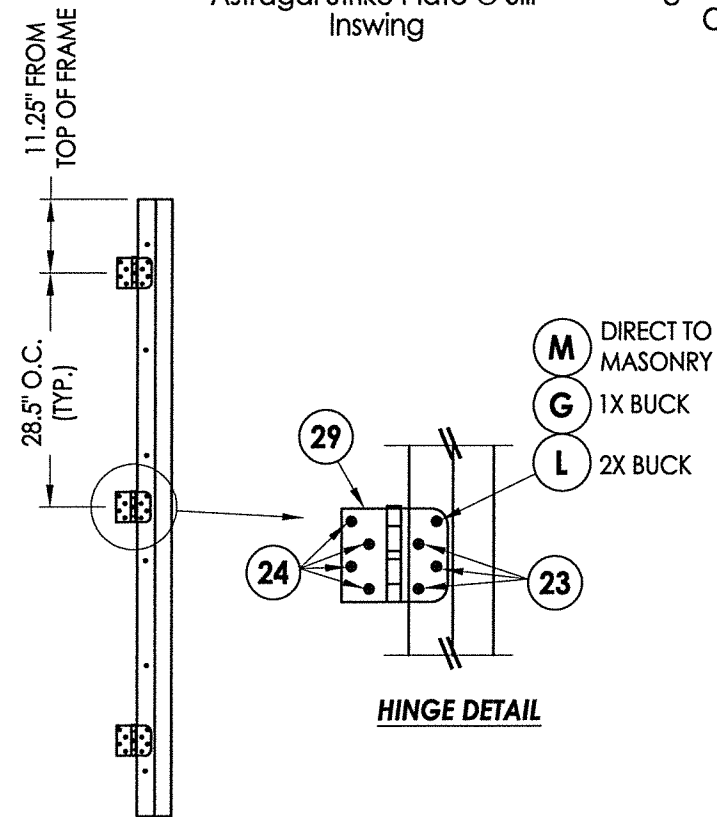
HINGE JAMB
